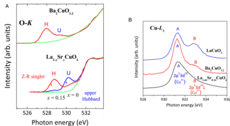
图2. 通过X射线吸收谱测得掺杂浓度。(A) Ba214 and LSCO [ x = 0 (blue) and 0.15 (red)]的氧K边吸收谱，U和H分别源于O1s芯能级至铜的上Hubbard带和掺杂空穴态，对应于 Cu^{2+} 态和 Cu^{3+} 态 (即Zhang Rice单态)。(B) Ba 2 CuO 3.2 、过掺杂的LSCO ( x = 0.34 )和LaCuO 3 的铜L边吸收谱，表明Ba 2 CuO 3.2 铜的价态处于超过掺杂状态。
