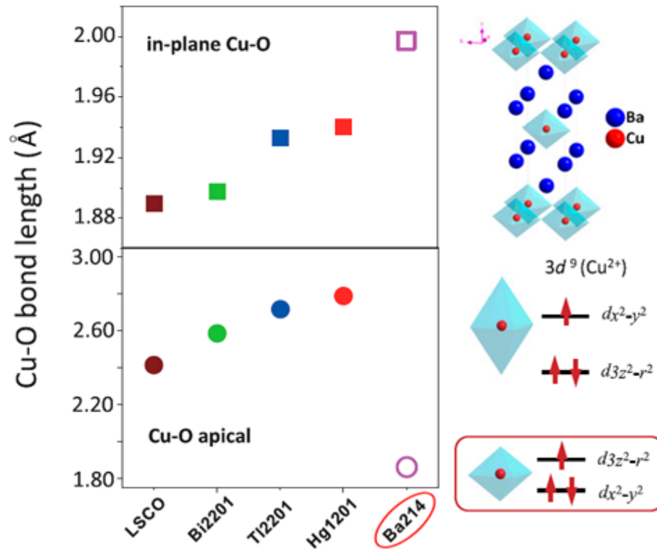
图1. 具有单层铜氧面结构的铜基超导材料的面内氧和顶角氧的铜氧键长、铜氧配位构型、铜的3d x^2-y^2 和 3z^2-r^2 轨道相对顺序。其中La系材料的顶角氧距离大于面内铜氧键长，呈现拉伸型铜氧六配位构型，导致 3dx^2-y^2 轨道居于 3dz^2-r^2 轨道之上。Ba214的面内铜氧键长大于顶角氧距离的压缩型铜氧配位构型，导致 3dz^2-r^2 轨道居于 3dx^2-y^2 轨道之上。
