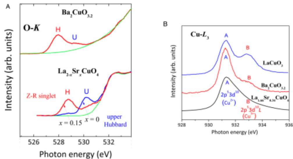
图2. 通过X射线吸收谱测得掺杂浓度。(A) \text{Ba}_2\text{CuO}_{3.2} and \text{La}_{2-x}\text{Sr}_x\text{CuO}_4 [x = 0 (blue) and 0.15 (red)]的氧K边吸收谱，U和H分别源于O1s芯能级至铜和掺杂空穴态，对应于 \text{Cu}^{2+} 态和 \text{Cu}^{3+} 态(即Zhang Rice单态)。(B) \text{Ba}_2\text{CuO}_{3.2} 、过掺杂的LSCO(x = 0.34)和 \text{LaCuO}_3 的铜L边吸收谱，表明价态处于超过掺杂状态。
