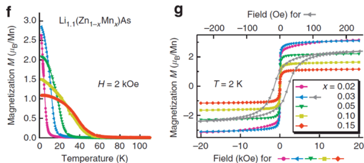
图2: \text{Li}_{1.1}(\text{Zn}, \text{Mn})\text{As} 的磁性随Mn掺杂量的演化, 在3%Mn含量即具有2.8Bohr磁子的饱和磁矩, 矫顽场约为300e.
