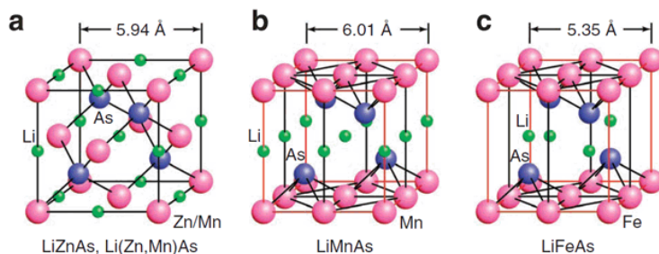
图1: (a) LiZnAs、(b) LiMnAs、(c) LiFeAs的晶体结构
